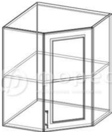
ШВУС-590 (ШxBxГ) 590x716x590 мм
