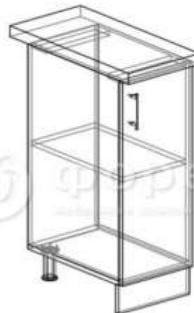
ШН-300 (ШxBxГ) 300x840x474 мм
