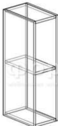
ШВБ-200 (ШxBxГ) 200x716x298 мм
