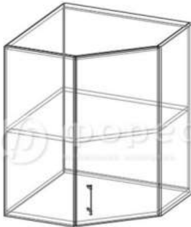
ШВУ-557 (ШxBxГ) 557x716x557 мм
