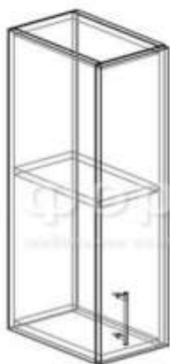
ШВ-200 (ШxBxГ) 200x716x314 мм
